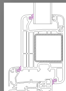
Seuil plat 40mm
