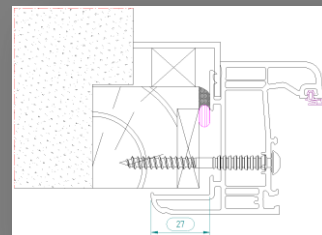
Dormant rénovation avec aile de 27mm
