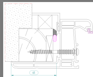
Dormant rénovation avec aile de 65mm
