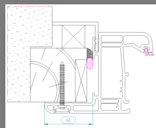
Dormant rénovation avec aile de 42mm
