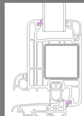
Seuil PMR 20mm
